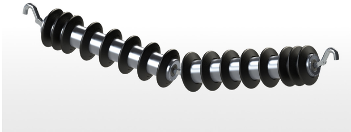
GHIRLANDA A 2 RULLI CON ANELLI 2-ROLL GARLAND WITH RINGS
